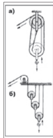
Рис.16. Поліспасти: а – кратний; б – ступеневий
