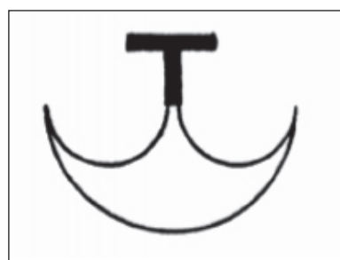
Рис. 23. Ніж «Арбелос»
