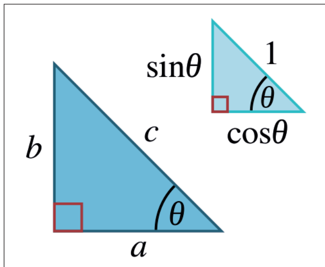
Рис. 7. Синус і косинус кута \theta
