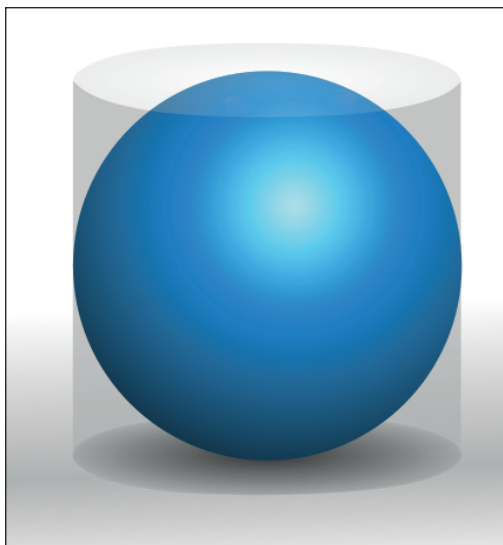
Рис.17. Циліндр і куля
