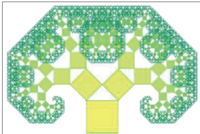
Рис. 8. Класичне дерево Піфагора
