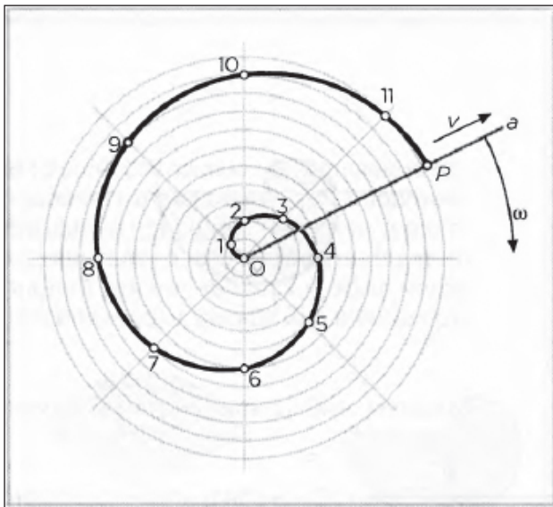
Рис. 36. Спіраль Архімеда
