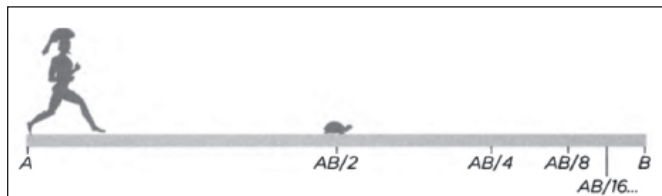
Рис. 22. Ахіллес і черепаха
