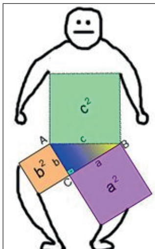
Рис. 4. «Піфагорові штани»
