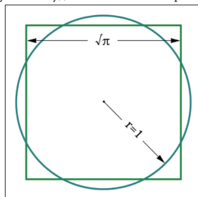
Рис.1. Квадратура круга
