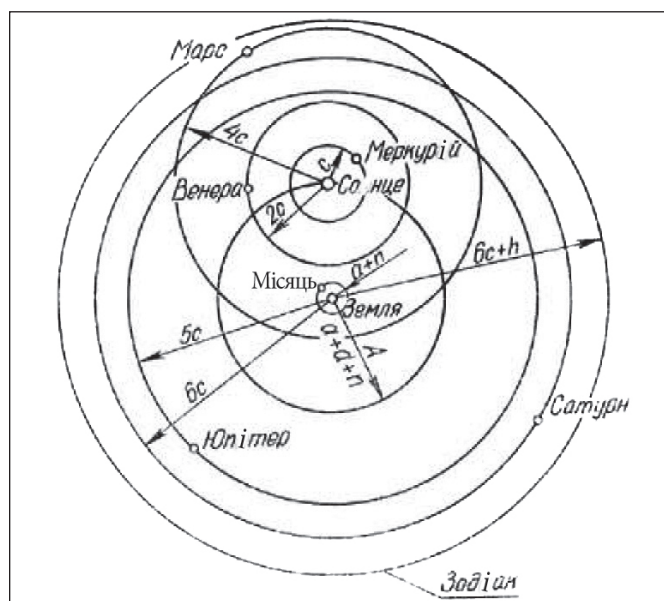
Рис. 35. Система світу Архімеда. Міжпланетні віддалі подані в міріадах стадій: a = 554 , d = 5081 , A = 5640 , c = 2027 , h = 2007 , n = 4
