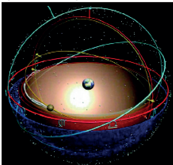
Рис. 34. Планетарій Архімеда
