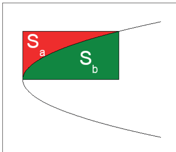
Рис.19. Площа сегмента параболи
