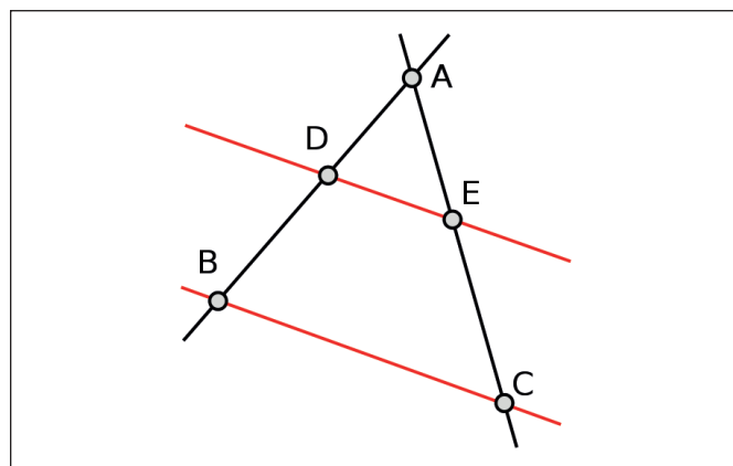
Рис.3. Теорема Фалеса
