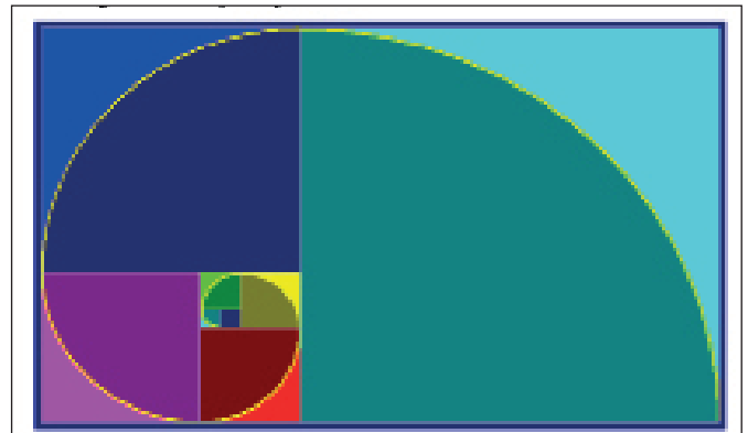
Рис.38. Логарифмічна спіраль
