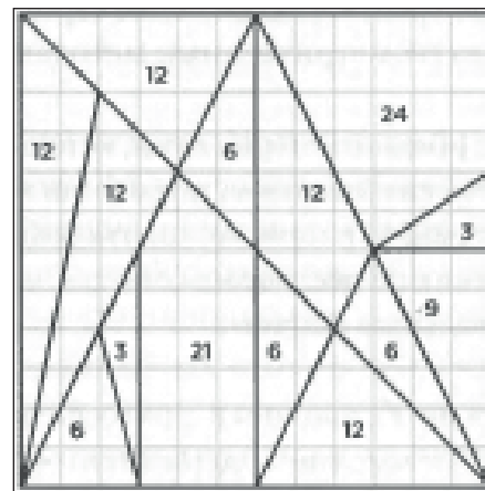
Рис. 27. «Стомахіон» Архімеда
