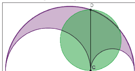
Рис. 24. Площа Арбелоса
